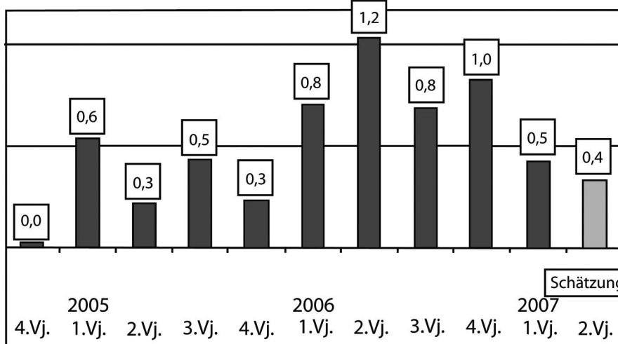
Arbeitstäglich und saisonbereinigtes reales Bruttoinlandsprodukt in Deutschland (Kettenindex)
